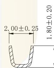
SEC D-D
