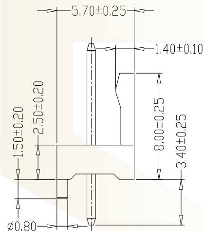
位置可定制 塑件带柱图视:
