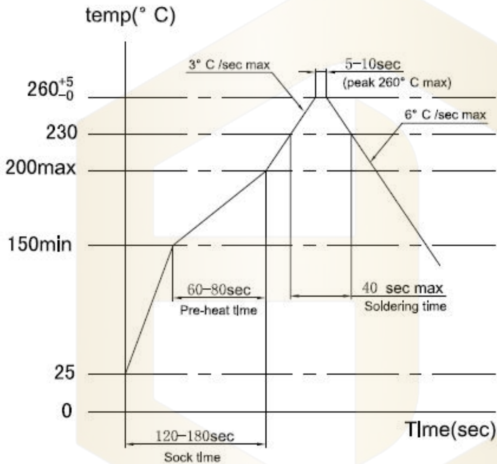
回流焊温度曲线图
