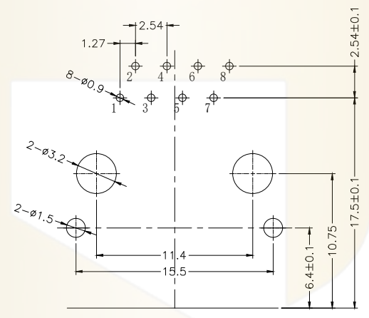
P. C. B参考图
