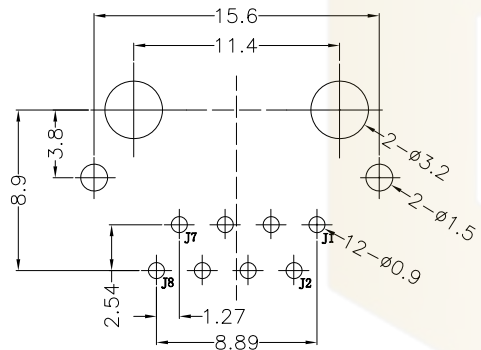
P. C. B参考图 (建议板后1.6mm)
