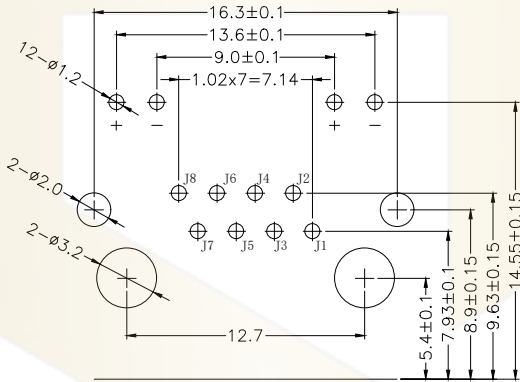
P.C.B参考图
