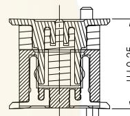
公、母座合高图
