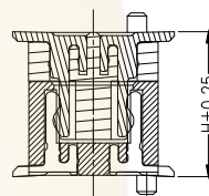
公、母座合高图
