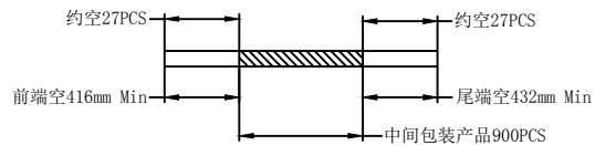
1.载带包装示意图
