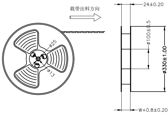
1.载带包装示意图
